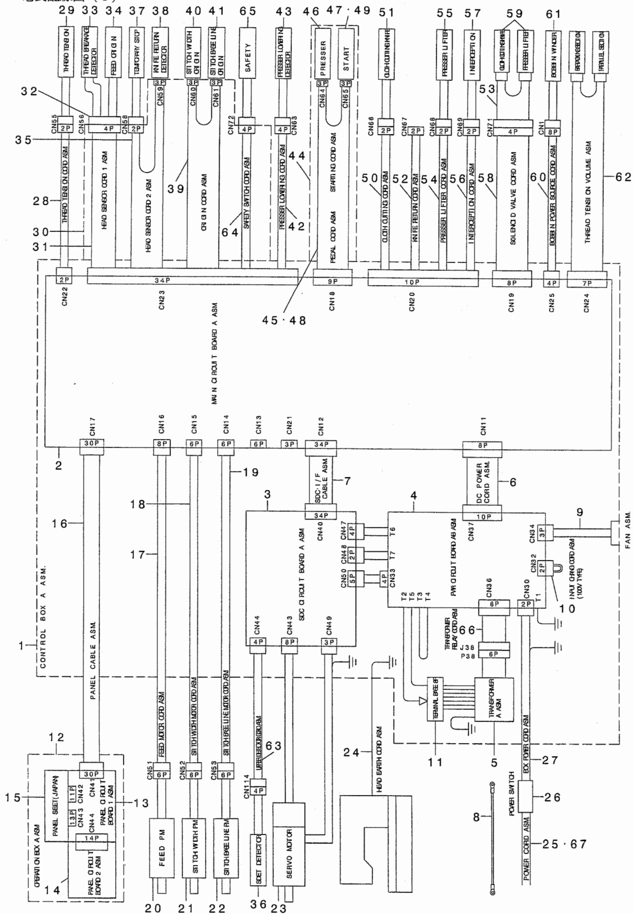
電装配線図 (1)
